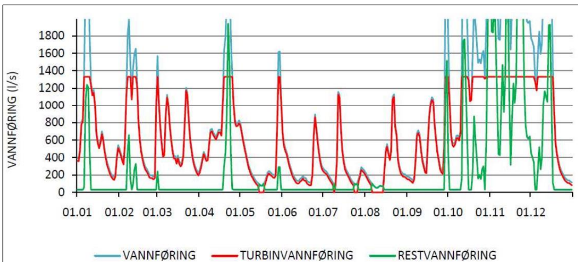
Figur V3. Vannføringsvariasjon i et vått år (2000) før (blå) og etter (grønn) utbygging.
